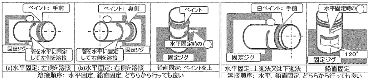
図4 薄肉管の固定方法と溶接姿勢
